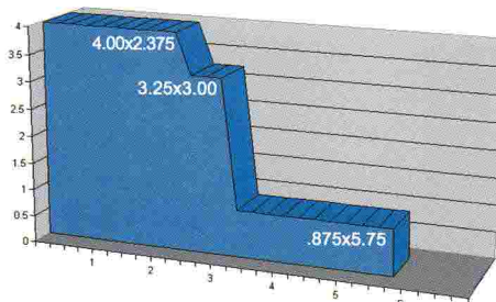
12" Blade
